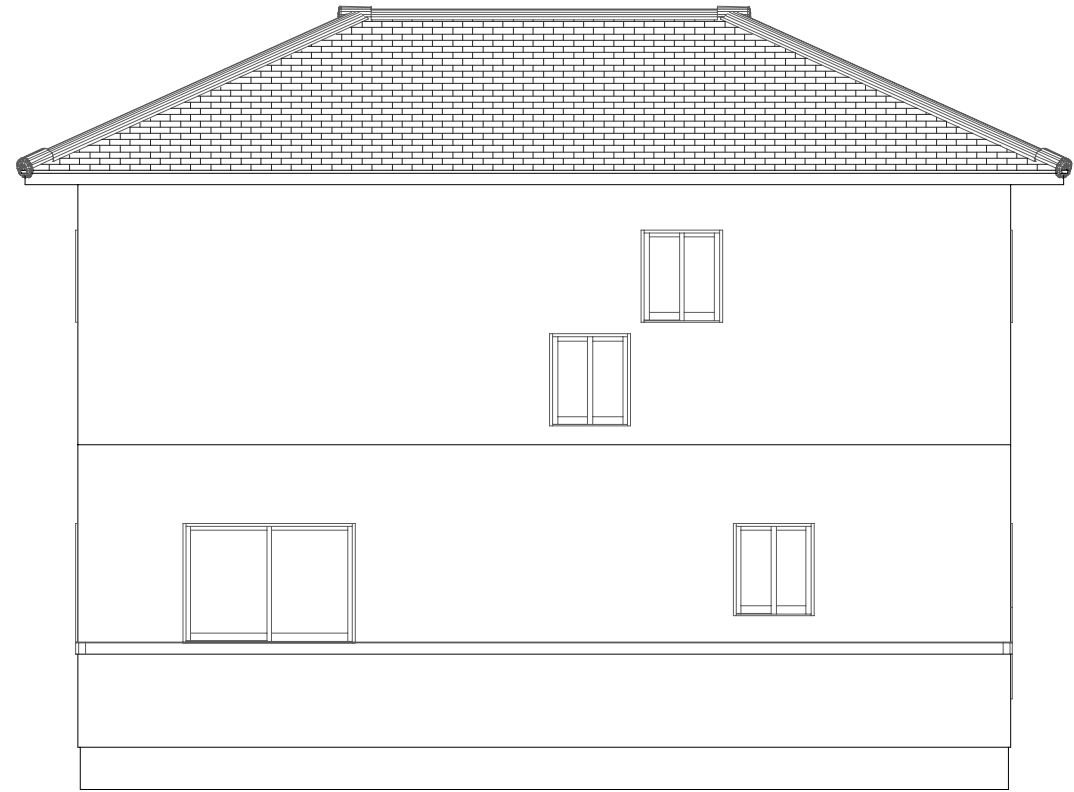
北侧立面图
