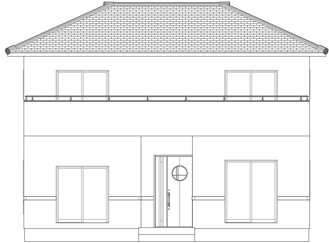
南侧立面图
