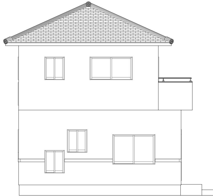
西侧立面图
